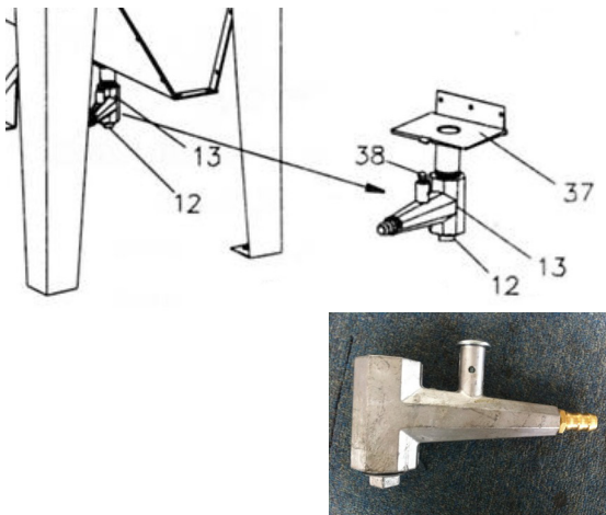
Abb. 5: Ventil Pos. 13
