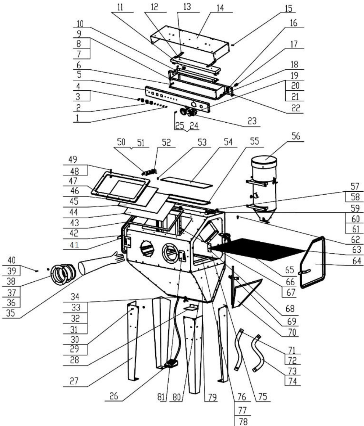
Abb. 8: Ersatzteilzeichnung SSK 2.5
